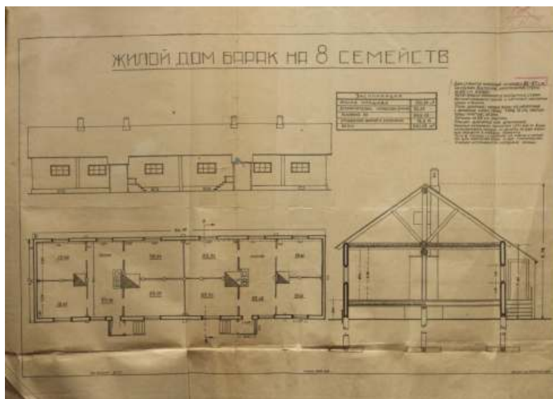
Схема жилого дома-барака на восемь семейств для спецпереселенцев. 1930-е гг. Из фондов ВОАНПИ.
